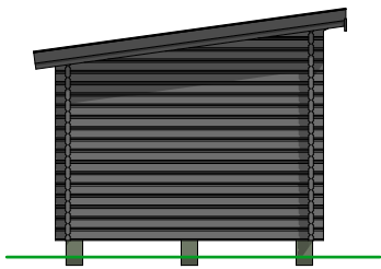
A1 Fasad 1:100
