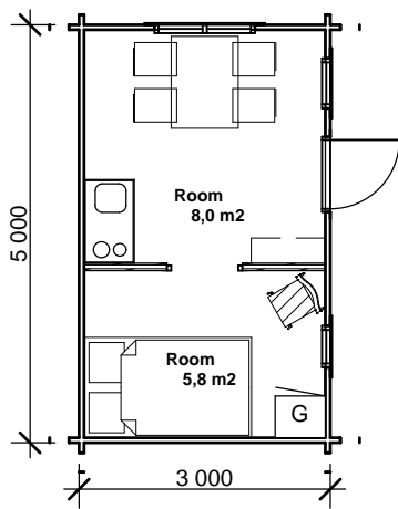
2. Plan 1:100
