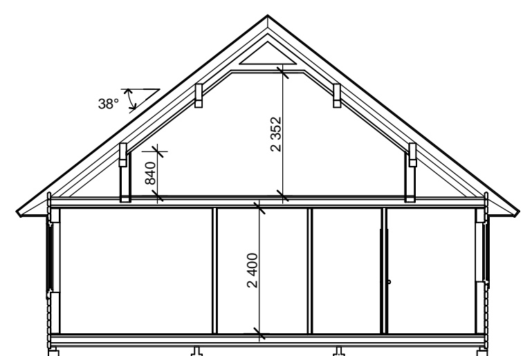
S1 1:100
