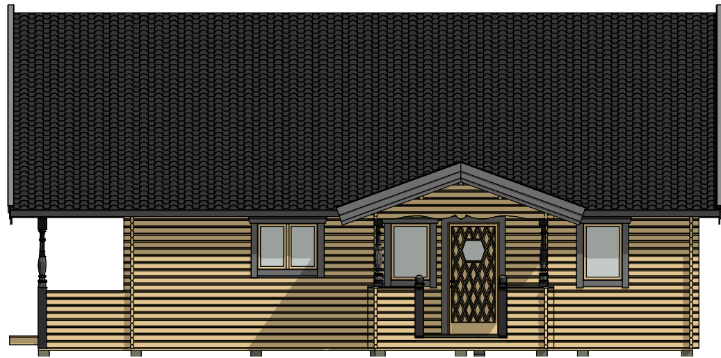
A1 Fasad mot 1:100
