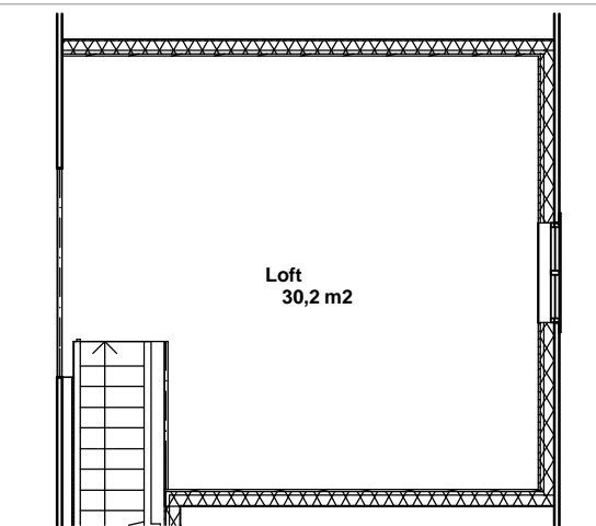
2. Plan loft 1:100
