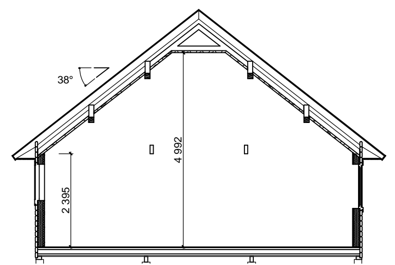
S3 1:100
