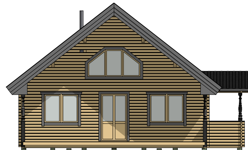
A4 Fasad mot 1:100
