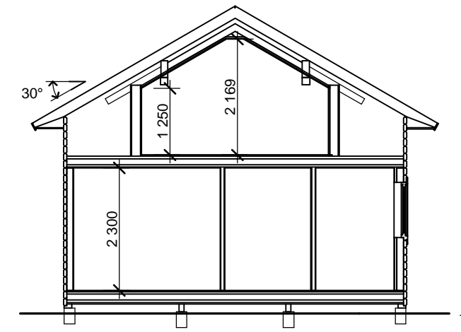
S1 1:100
