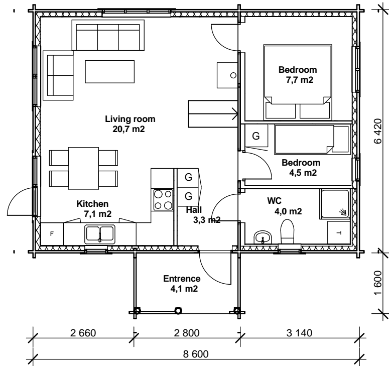
1. Plan 1:100
