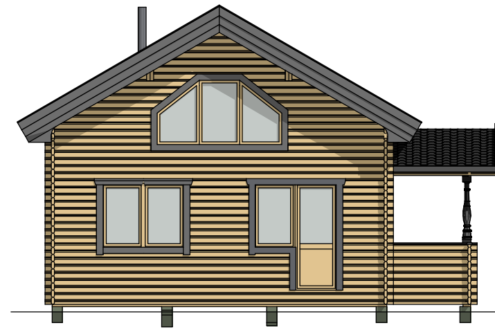
A4 Left view 1:100
