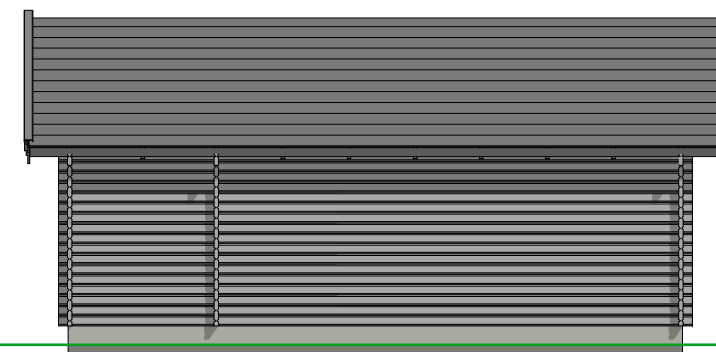
A1 Fasad 1:100
