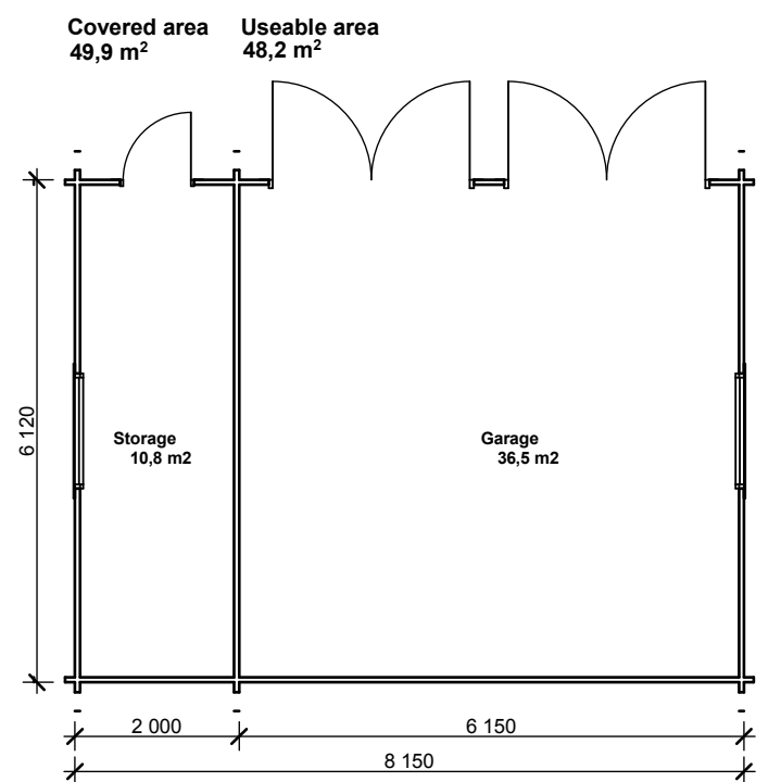
2. Plan 1:100
