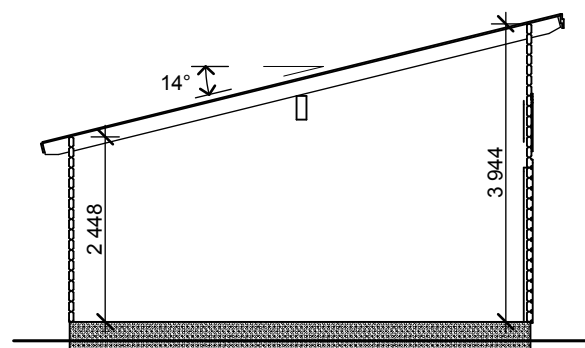
S1 1:100
